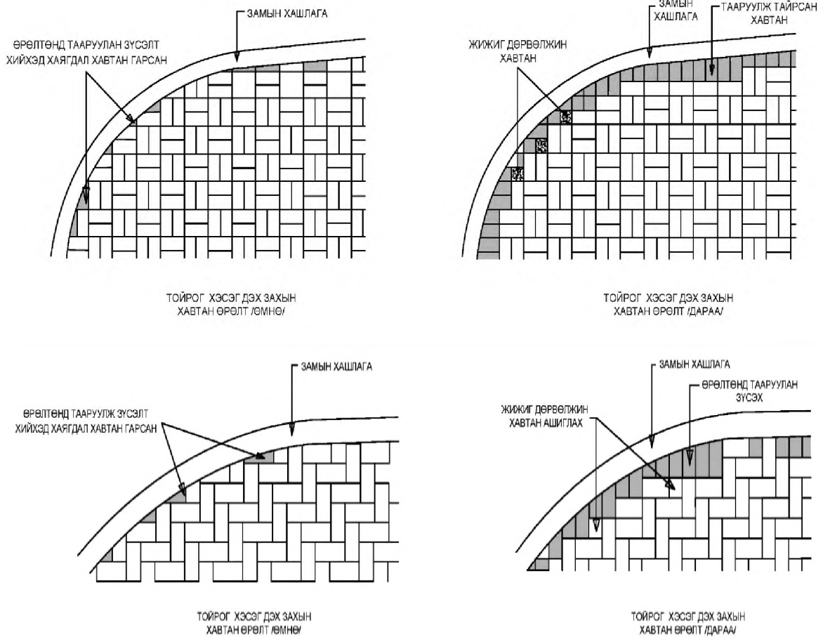
Зураг 16.2. Хавтан өрөх технологийн алдаа болон залруулга
