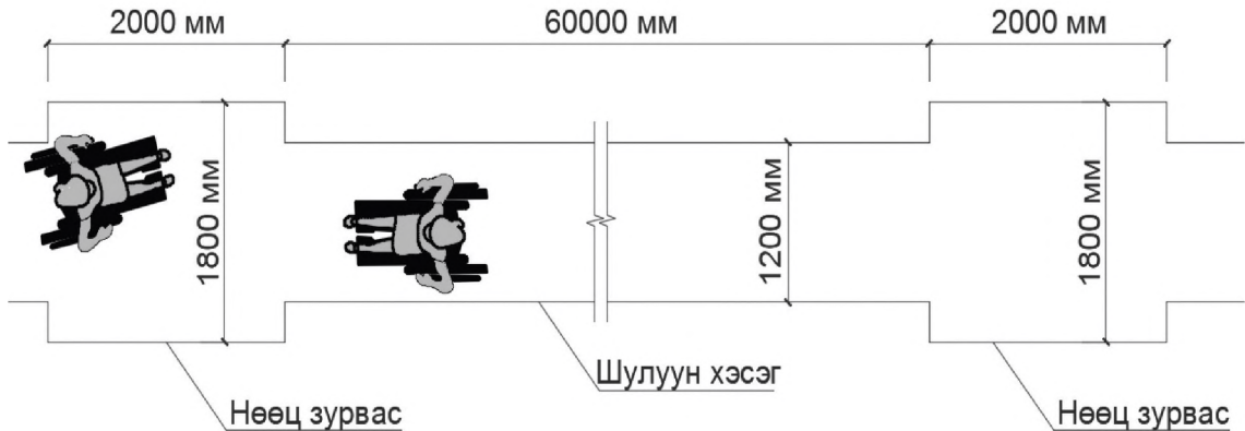
Зураг 4.6. Явган хүний замын нөөц зурвас байгуулах (ЖИШЭЭ)
