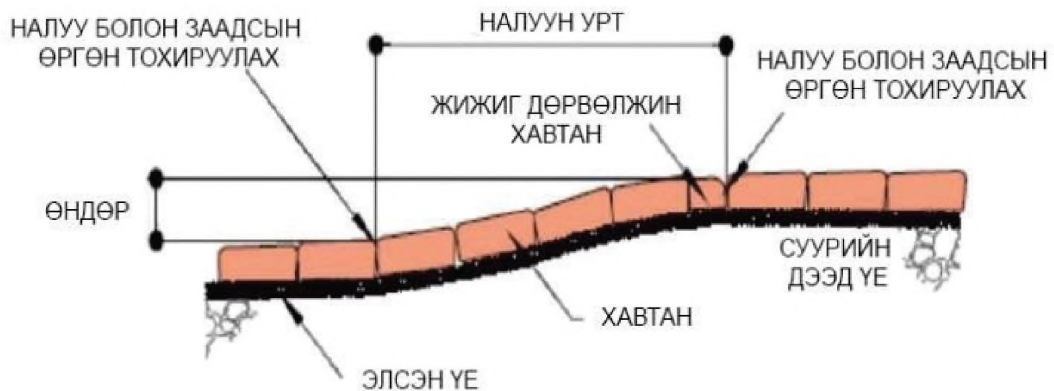
Зураг 16.13. Налуу газар хавтан өрөх технологи
