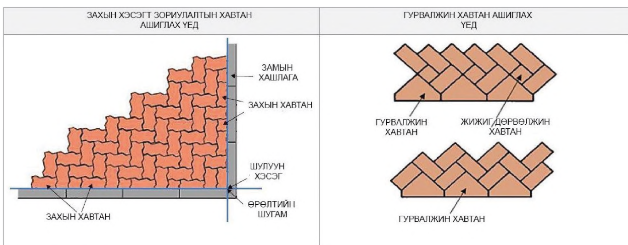
Зураг 15.4. Зах ирмэгийн зориулалттай хавтан өрөх (ЖИШЭЭ)
