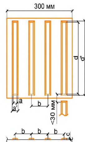
Зураг 6.7. Чиглүүлэх хавтан
