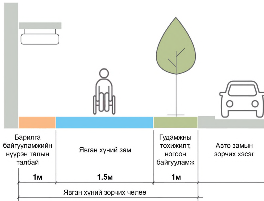
Зураг 4.4. Явган хүний зорчих чөлөөний хэсгүүдийн хамгийн бага утга
