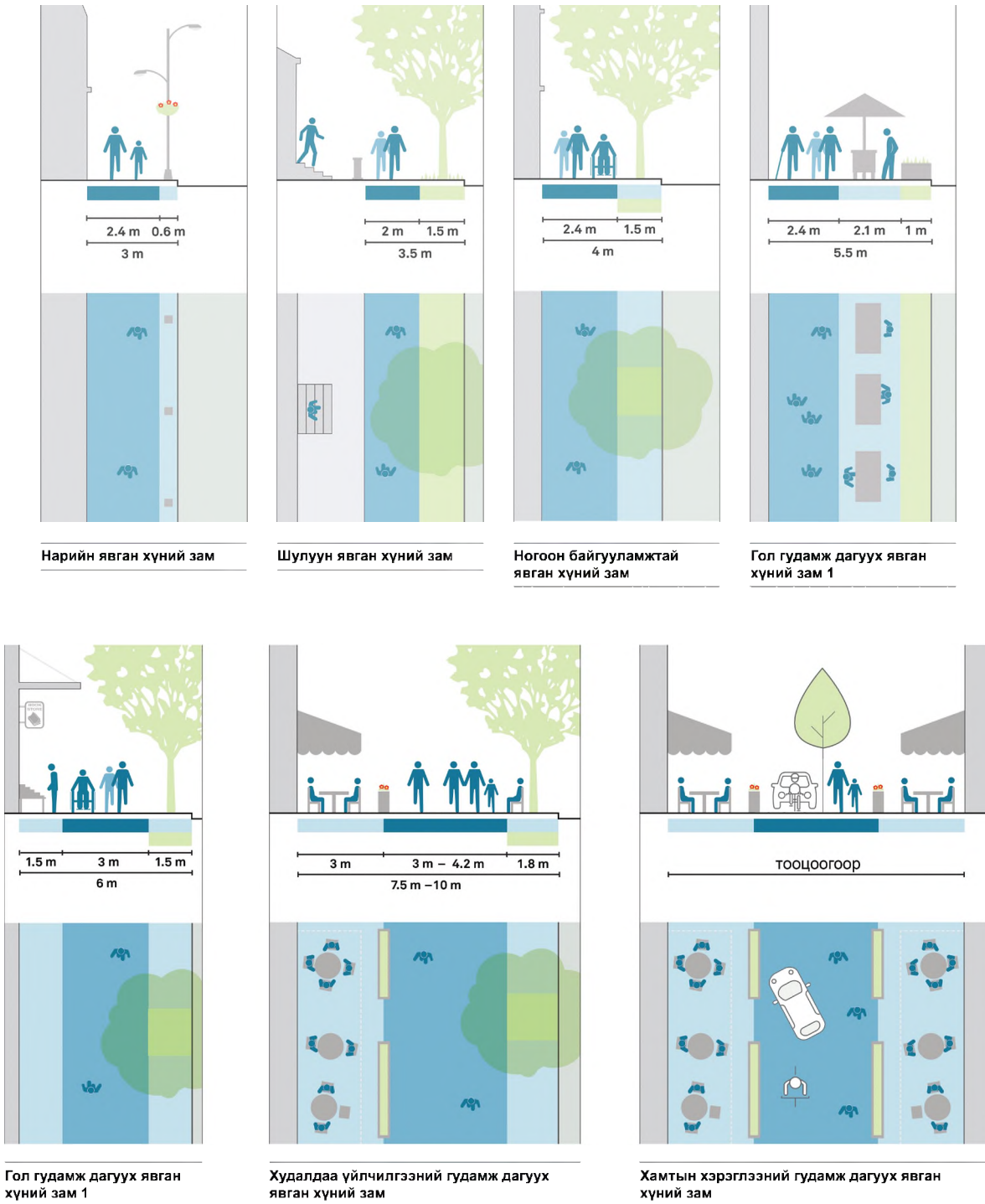
Зураг 4.5. Явган хүний замын хэмжээс (ЖИШЭЭ)
