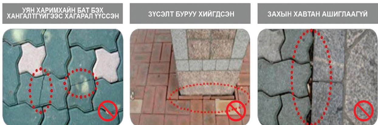
Зураг 15.2. Хавтанг буруу өрсөн (ЖИШЭЭ)
