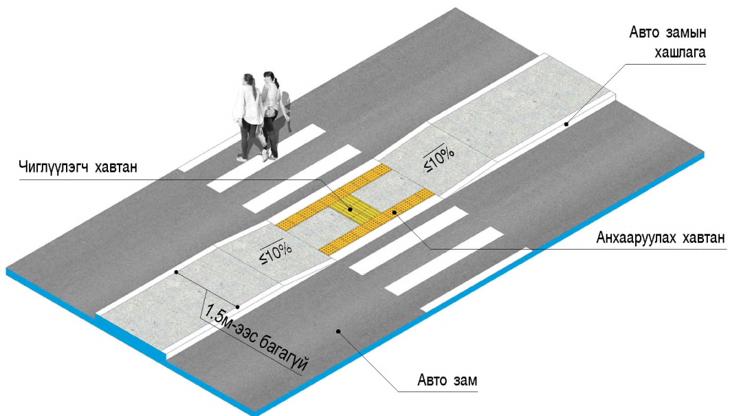
Зураг 7.2. Нэг чиглэлийн гарц
