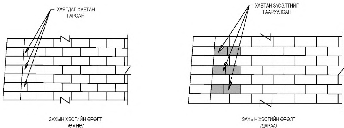
Зураг 16.1. Хавтангийн хөндлөн өрөх технологийн алдаа болон залруулга
