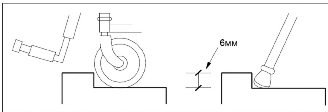
Зураг 6.3. Явган хүний замын гадаргуугийн түвшний өөрчлөлт
