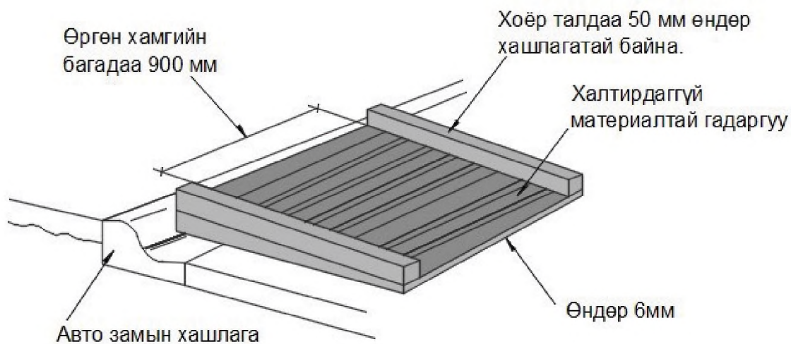
Зураг 9.6. Түр налуу замд тавих шаардлага
