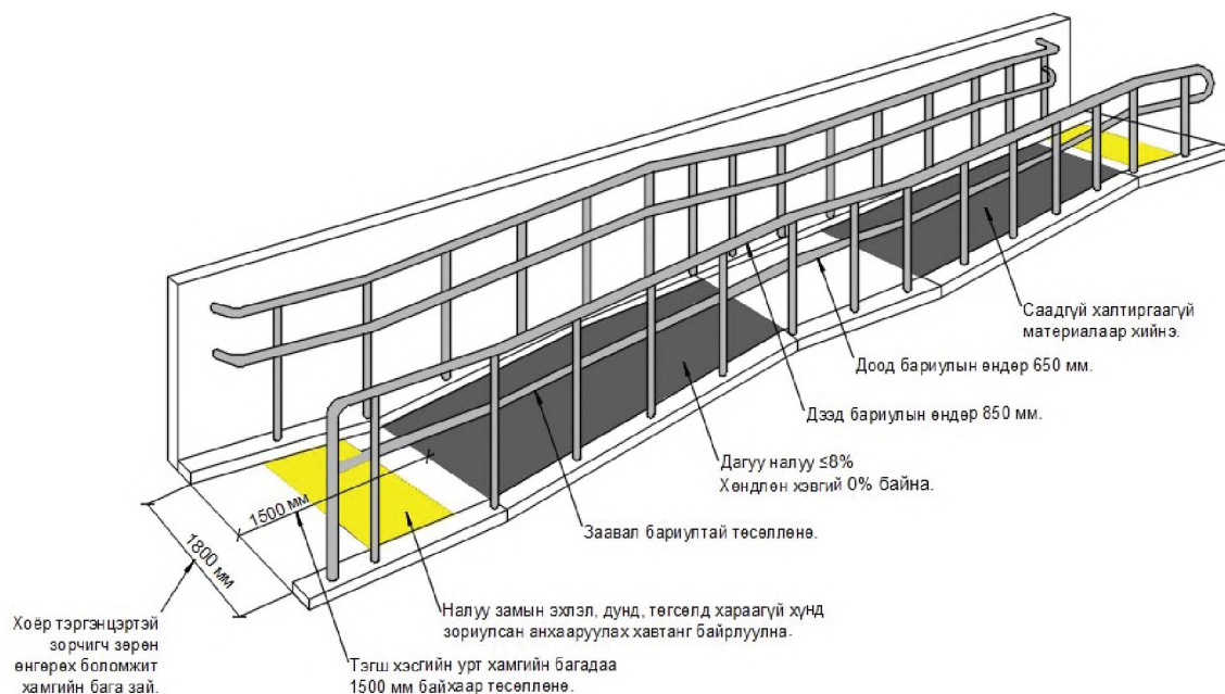
Зураг 9.3. Налуу замын шаардлага (ЖИШЭЭ)
