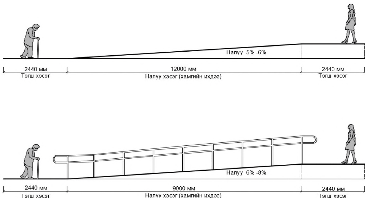
Зураг 5.2. Дагуу налуу, хөндлөн хэвгий
