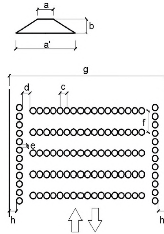
Зураг 7.8. Чиглүүлэгч шулуун
