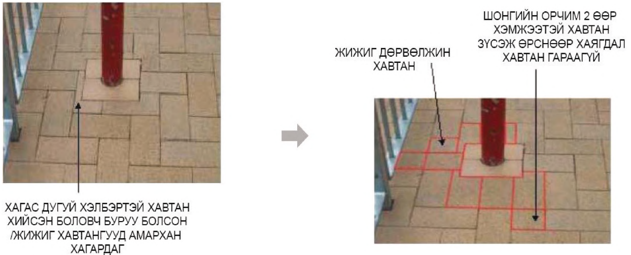
Зураг 16.6. Хагас дугуй хэлбэртэй хавтан өрөх технологийн алдаа болон залруулга
