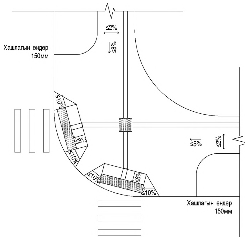
Зураг 7.5. Холимог перпендикуляр гарц
