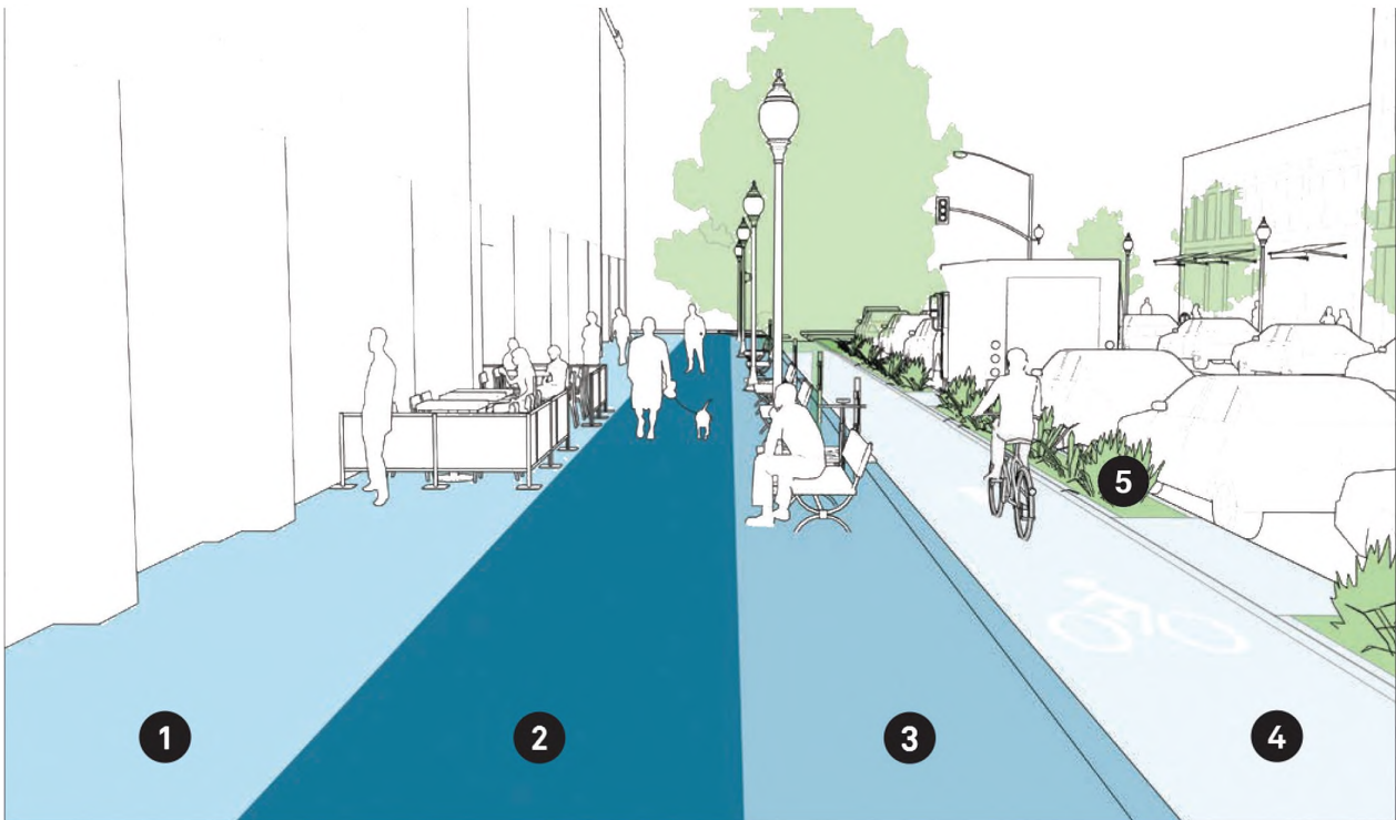
Зураг 4.3. Явган хүний замын зорчих чөлөө
