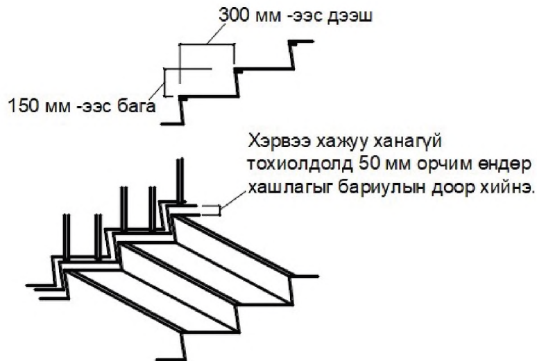
Зураг 9.1. Шатны хэмжээ
