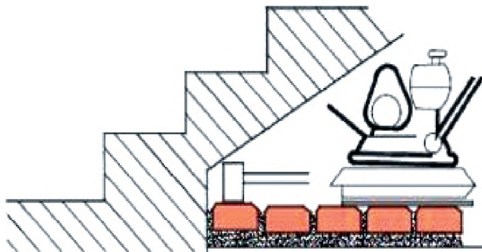
Зураг 14.4. Хавтант хучилтыг нягтруулж буй байдал
