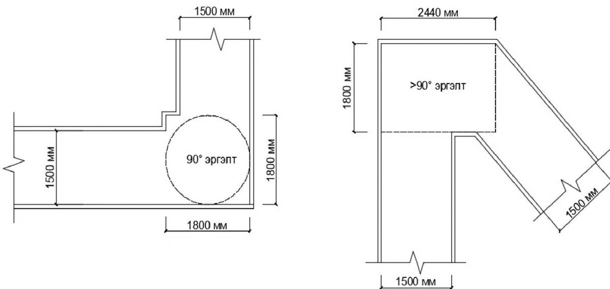
Зураг 5.4. Явган хүний замын эргэлттэй хэсгийн орон зайн зөвшөөрөх хэмжээ
