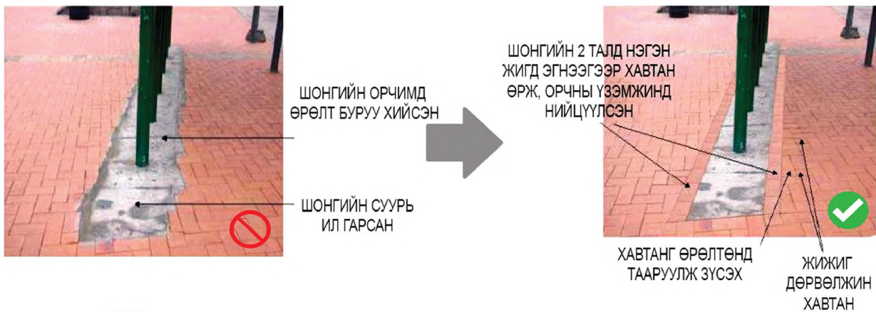
Зураг 16.7. Шонгийн ойр орчим хавтан өрөх технологийн алдаа болон залруулга
