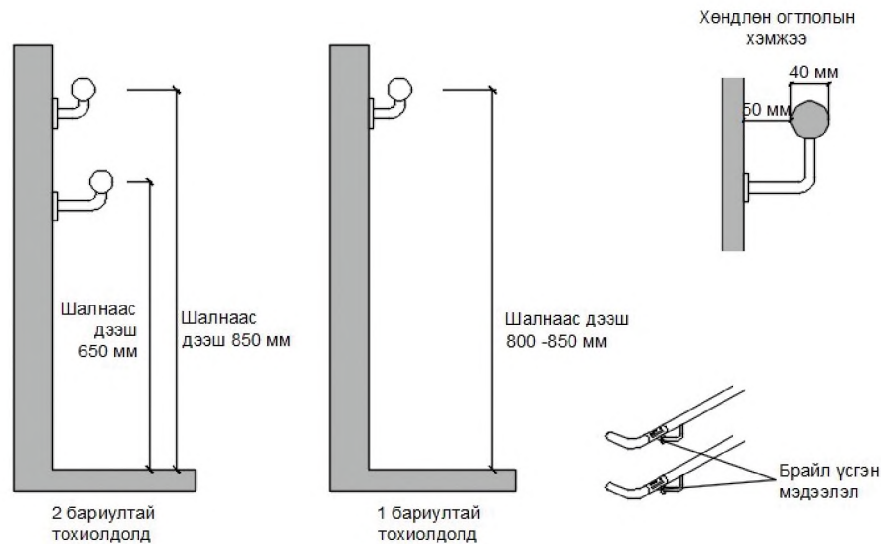
Зураг 9.2. Шатны бариул
