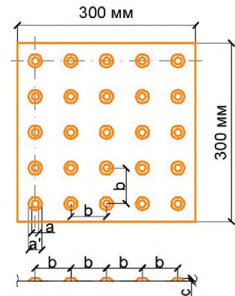
Зураг 6.6. Анхааруулах хавтан
