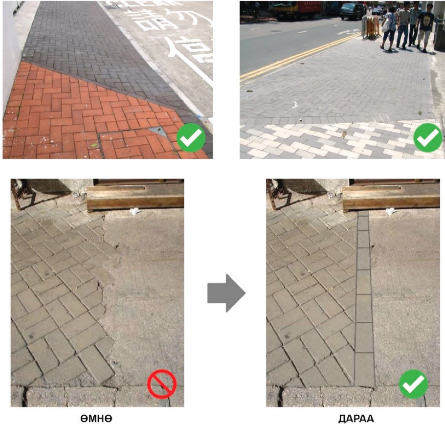
Зураг 16.4. Өөр төрлийн хавтантай нийлэх хэсгийн өрөлт
