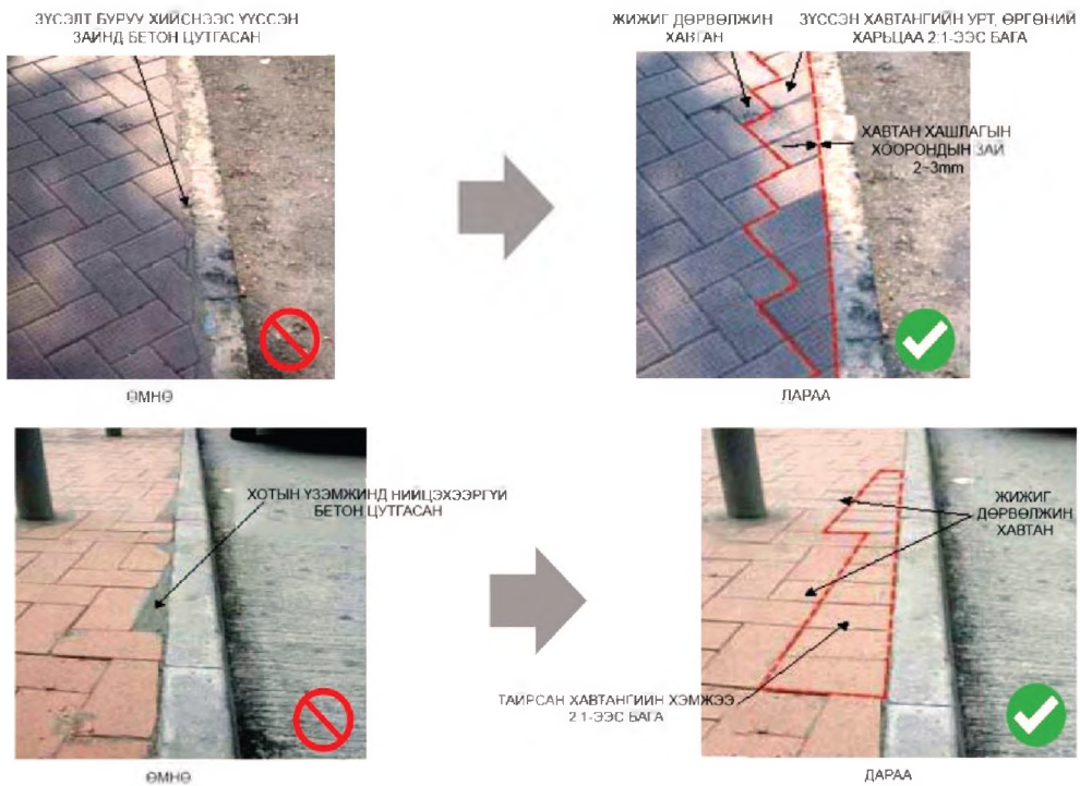
Зураг 16.3. Хашлаганы ойролцоо хавтан өрөх технологийн алдаа болон залруулга
