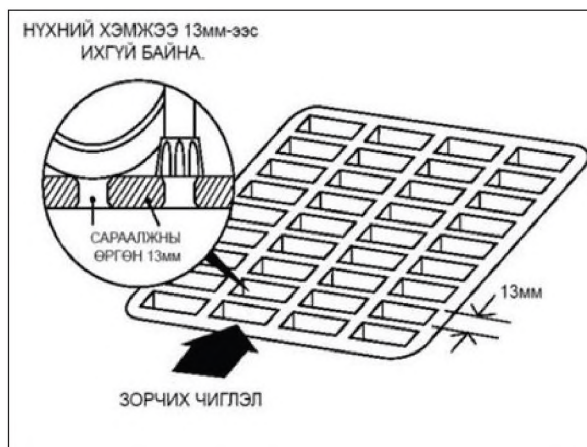
Зураг 6.4. Сараалжин таг
