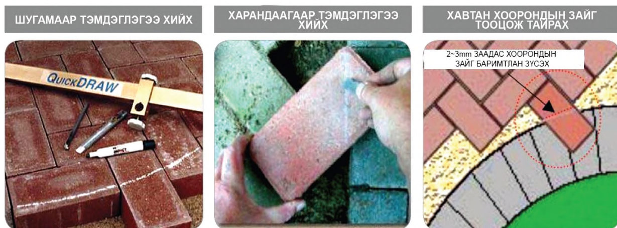
Зураг 15.7. Зүсэх шугам тэмдэглэх
