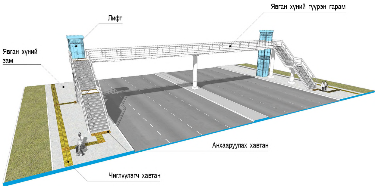
Зураг 7.4. Явган хүний гүүрэн гарц
