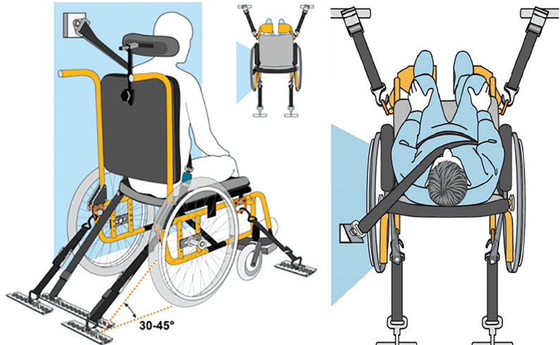
Зураг 5.7. Автобусанд тэргэнцрийг түгжсэн байдал
