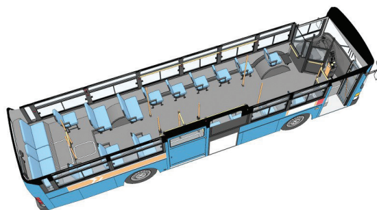
Зураг 6.2. Үйлчилгээний танхимын харагдах байдал
