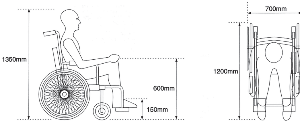
Зураг 6.8. Тулгуур эрхтний хөгжлийн бэрхшээлтэй иргэн тэргэнцэртэй зорчих зай
