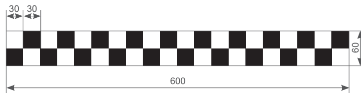
Зураг 6.1. Нийтийн такси таних “цоохор” тэмдэг
